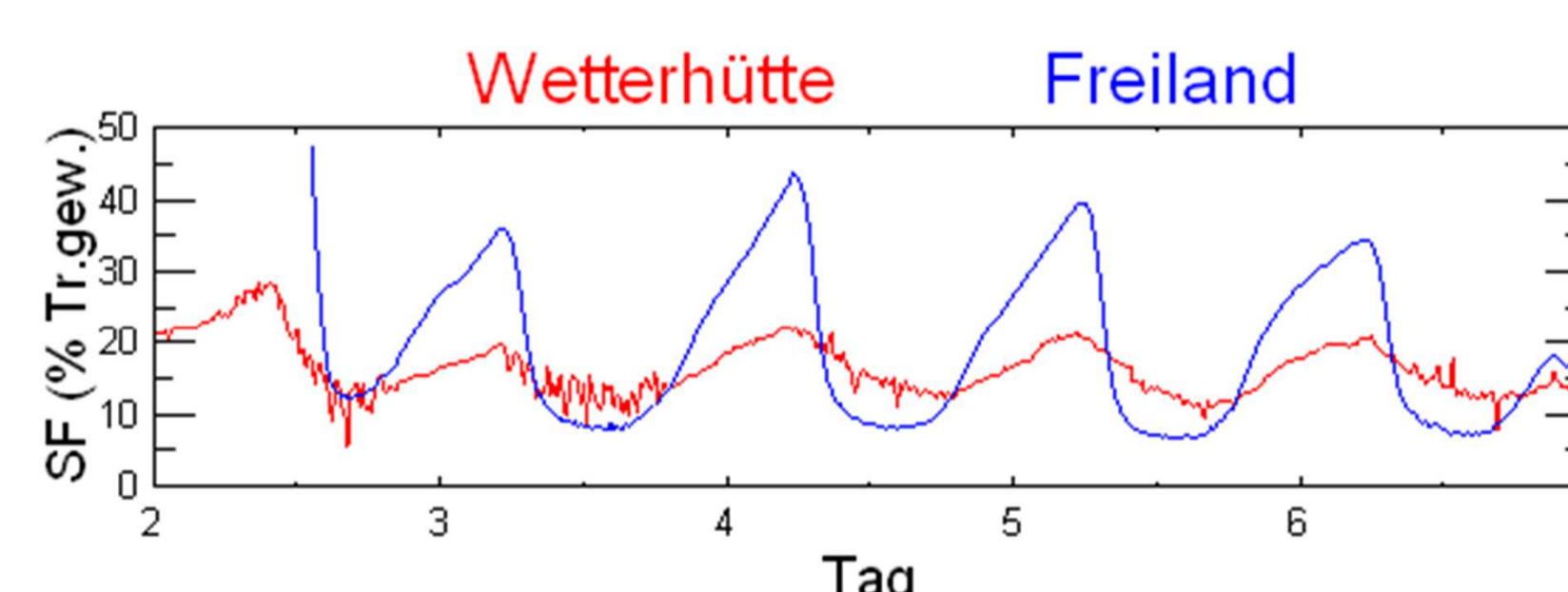
Abb. 3: Tagesgang des gemessenen Feuchtegehaltes vergilbten Grasses (Braunschweig, Juni 2010).
